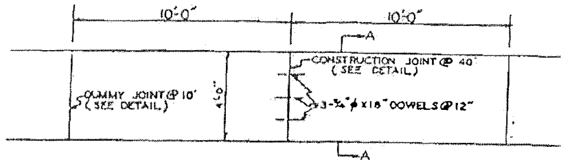
PLAN SCALE: 1/4" = 1'-0"
